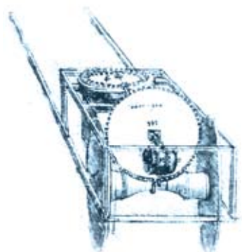
Измеритель пути «Атлантический кодекс», лист 1br примерно 1504 г.
